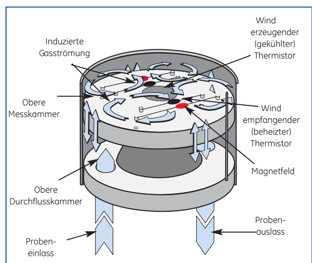
Strömungsschema der thermoparamagnetischen Sauerstoffmesszelle des XMO2. Die paramagnetischen Eigenschaften von Sauerstoff sorgen dafür, dass sich ein sauerstoffhaltiges Gas innerhalb des Magnetfeldes bewegt. Die Gasbewegung erzeugt einen „Magnetischen Wind“, der von den Thermistorpaaren aufgenommen wird. Die Sauerstoffkonzentration und die Trägergaskompensation werden durch den Mikroprozessor des Transmitters bestimmt.
